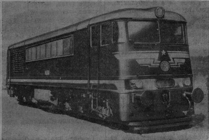
Чехословацкая Республика. Новый электровоз Т-698, изготовленный на заводе ЧКД-Соколово в Праге. Он предназначен для вождения как скоростных пассажирских, так и товарных поездов. Максимальная скорость 120 километров в час. Электровоз весит 107 тонн. Фото Чехословацкого телеграфического агентства.
