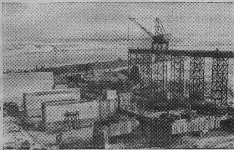
Недалеко от Ленинабада, в урочище Кайраккум, сооружается самая крупная в Средней Азии гидроэлектростанция. На снимке: строительство Кайраккумской ГЭС на реке Сыр-Дарье. Фото И. Кургана.
