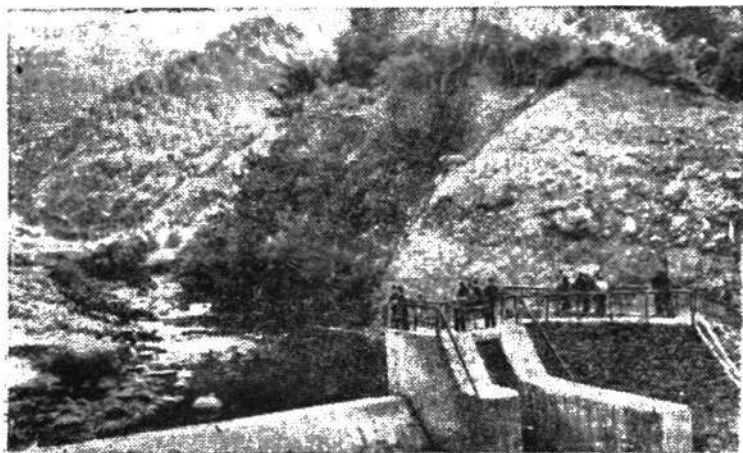
Аджарская АССР. Недавно пущена в эксплуатацию межколхозная гидроэлектростанция, построенная на реке Кинтриши в Кобулетском районе. Мощность ее—550 киловатт. Станция будет обслуживать восемь колхозов.
