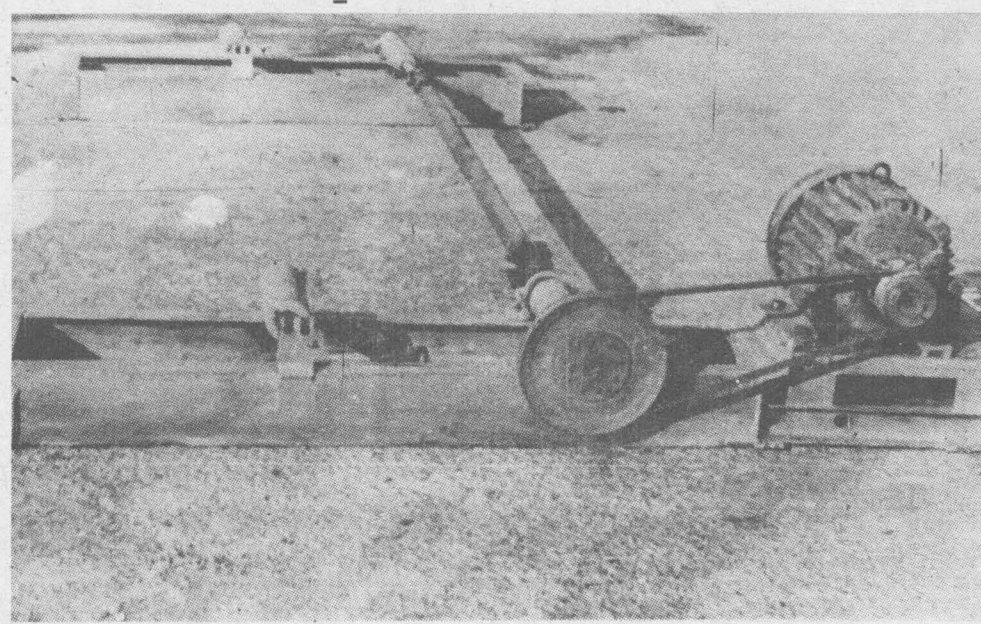
Стенд для обкатки сеялок.
