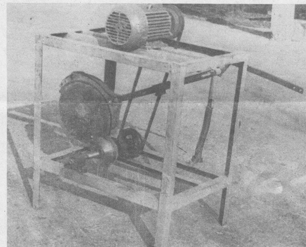
Стенд для обкатки сошников сеялок.
