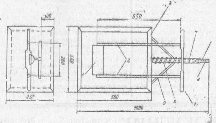
Приспособление для регулировки нажимных пружин сошников сеялки: 1 — груз; 2 — направляющие стержни; 3 — подставка; 4 — штанга; 5 — стойка; 6 — крючок; 7 — пластина; 8 — проверяемая пружина; 9 — подкосы.
