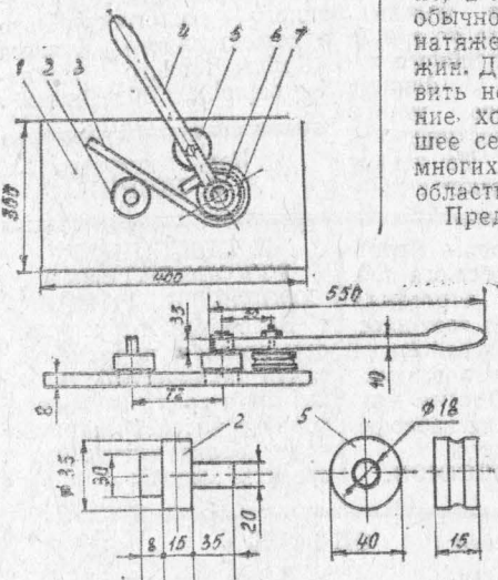
Приспособление для изготовления восьмерок в борон: 1 — плита; 2 — ось; 3 — пружина; 4 — ручка; 5 — ролик; 6 — втулка; 7 — ось.
