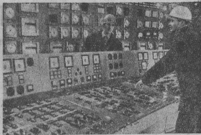
ДОНЕЦКАЯ ОБЛАСТЬ. Уг- легорская ГРЭС — пусковая стройка девятой пятилетки. НА СНИМКЕ: машинисты Л. В. Яковлев и В. Ф. Литов- кин у блочного щита управле- ния.
