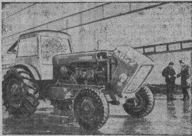
Недавно экспериментальным цехом будапештского завода «Красная звезда» изготовлен образец нового шестилитрового трактора типа «Дутра-4652». Мощность двигателя машины — 90 лошадиных сил. Фото МТИ-ТАСС.
