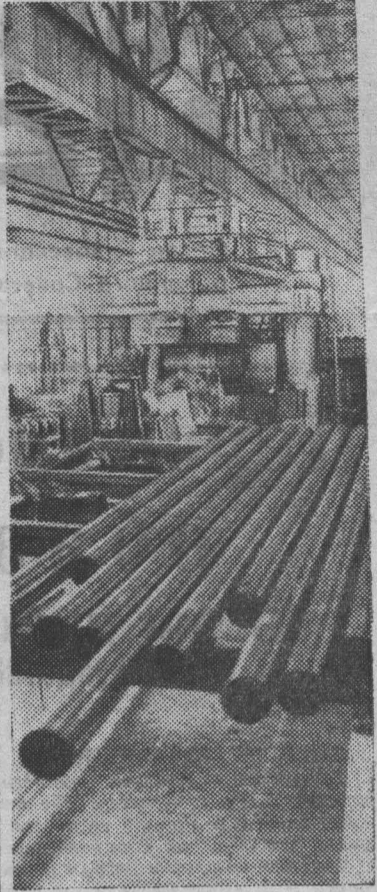
Коллектив Челябинского трубного завода начал промышленное освоение нового стана холодной прокатки труб «250». Он будет производить трубы диаметром 100—250 мм, высокой прочности, с зеркальной наружной и внутренней поверхностью.
