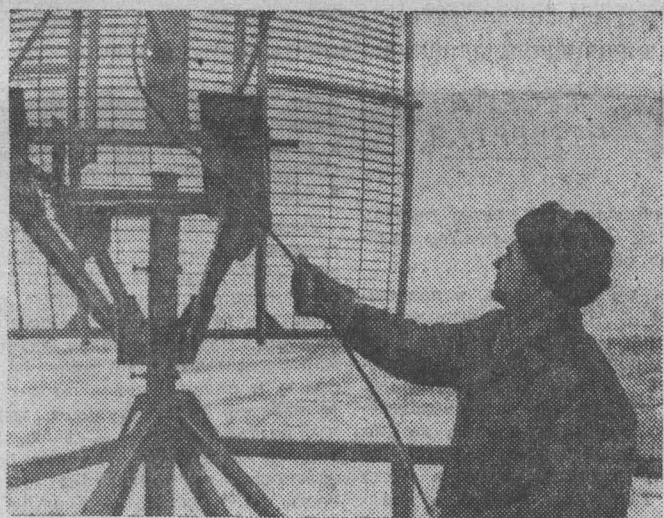
Запорожская область. Этот снимок сделан на высоте 38 метров. Электромеханик Михайловской районной конторы связи В. Площ проверяет направленную антенну. Недавно в районном центре Михайловке закончен монтаж новой радио-релейной линии, которая обеспечила связь района с Мелитополем и Днепрорудным. Фотохроника ТАСС.
