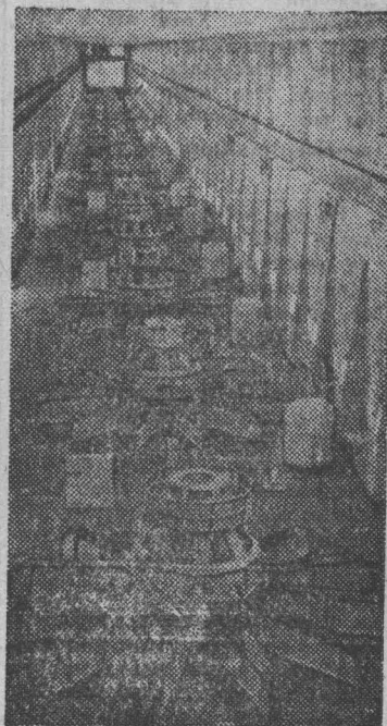
На днях Государственная комиссия приняла крупнейшую в мире Братскую гидроэлектростанцию в промышленную эксплуатацию с оценкой «отлично». ГЭС уже выработала более 60 миллиардов киловатт-часов электроэнергии. НА СНИМКЕ: машинный зал гидроэлектростанции. Фотохроника ТАСС.
