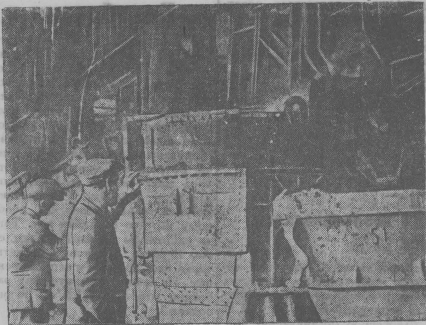
На снимке: выпуск стали на 4-й мартеновской печи.
