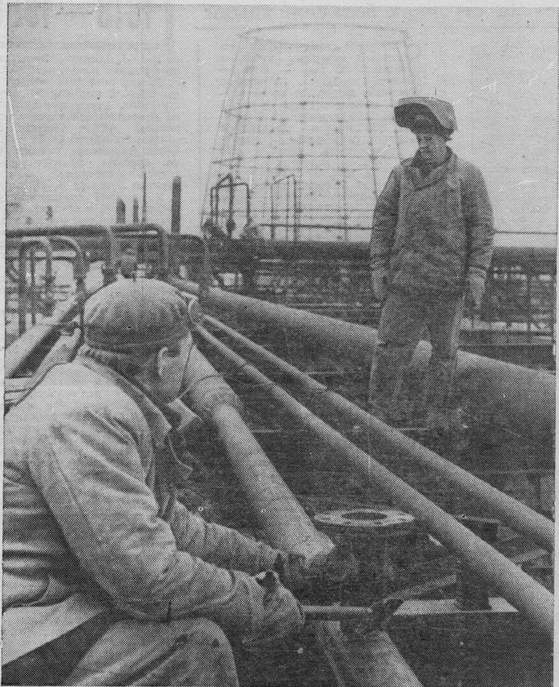
НА МОНТАЖЕ ТЕПЛОТРАССЫ.
