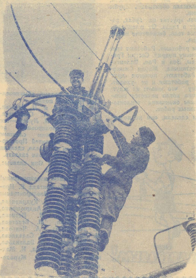
На снимке: электрики Лев Шефер и Сергей Фаронов из бригады т. Гусева устанавливают масляные раз'единители ОРУ-220. Это—хорошие ребята!
