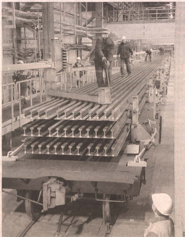
■ 100-метровые рельсы – гордость Кузбасса.
