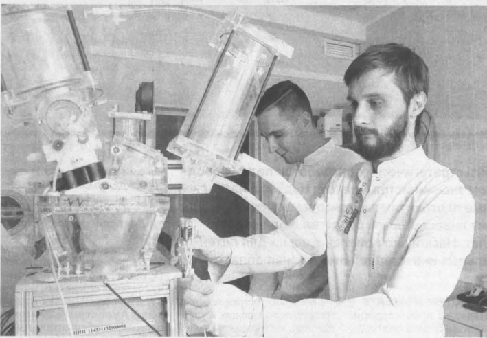
■ Стенд для испытания биопротезов в НИИ КПССЗ. Фото Федора Баранова.
