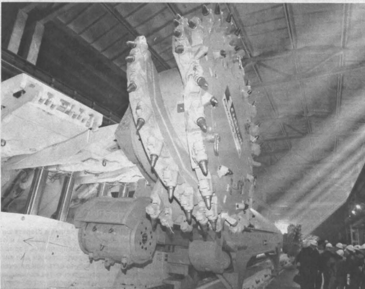
Комбайн Eickhoff SL 900.
