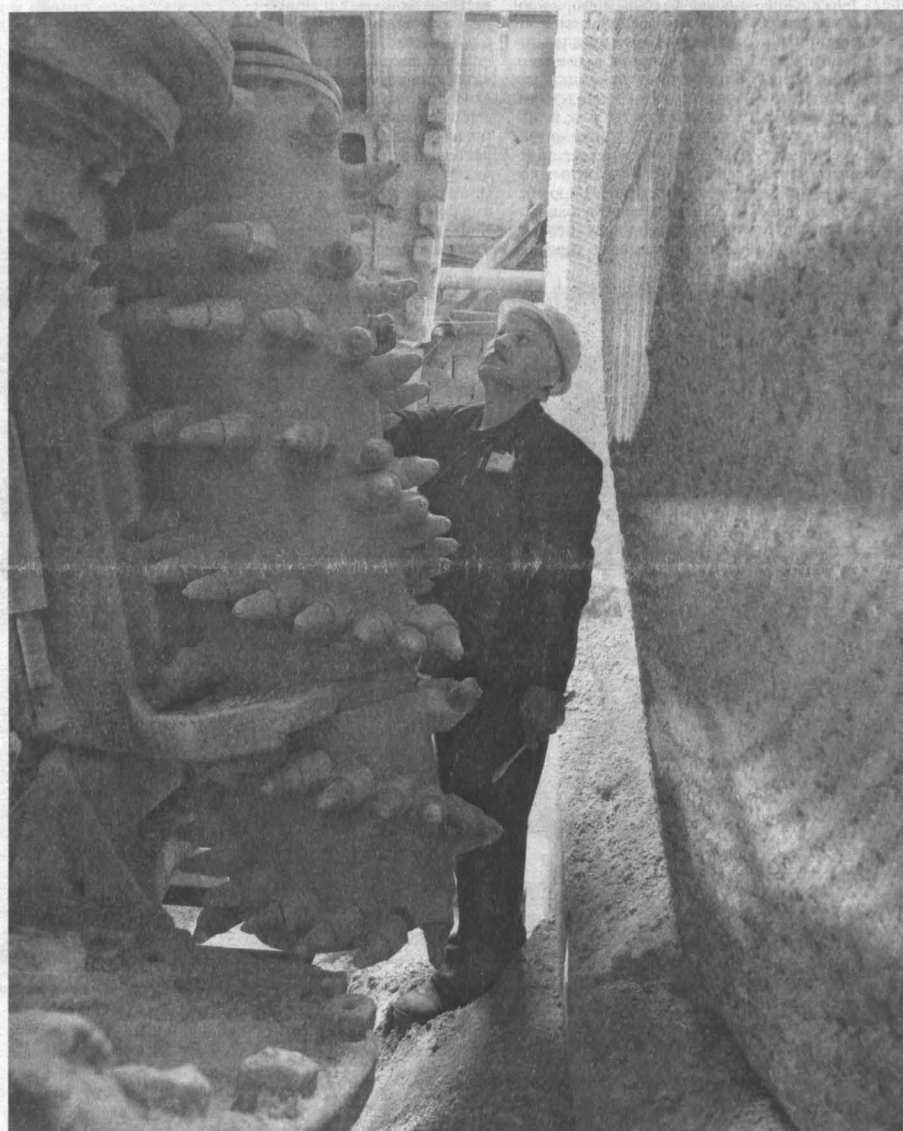
Геоход может работать в трёх плоскостях, а уникальность его — в режущей части, напоминающей обыкновенный саморез. Фото Сергея Гавриленко.
