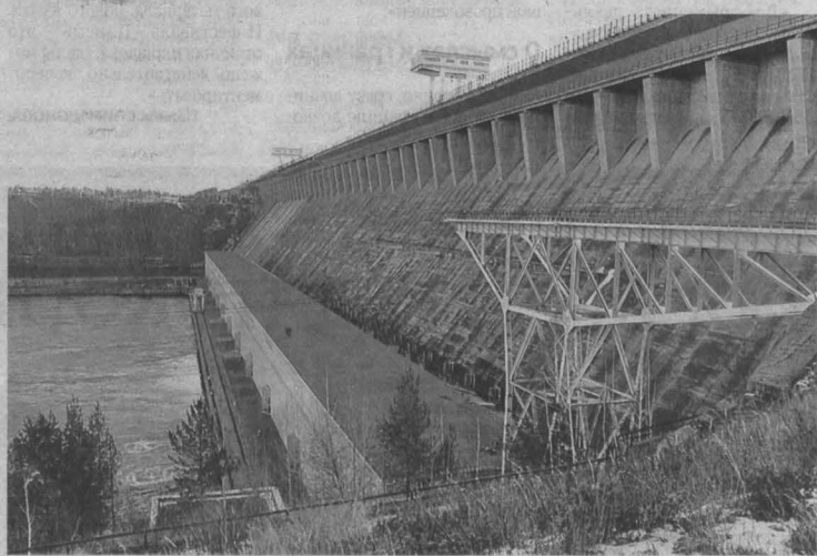
Братская ГЭС.
