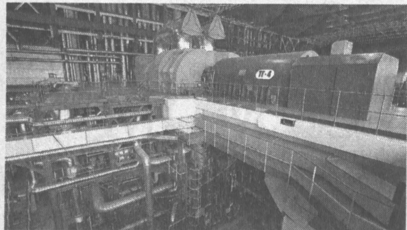
Реконструированная турбина в Белове. Фото Сергея Гавриленко.
