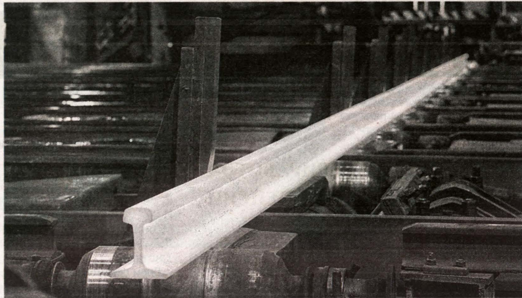
На ЗСМК в Новокузнецке начато промышленное производство 100-метровых рельсов по технологии дифференциации: верхняя часть закаляется больше, нижняя меньше, а средняя остается сырой. Это делает рельс пластичным, обеспечивая тем самым мягкость и бесшумность хода железнодорожных составов.
