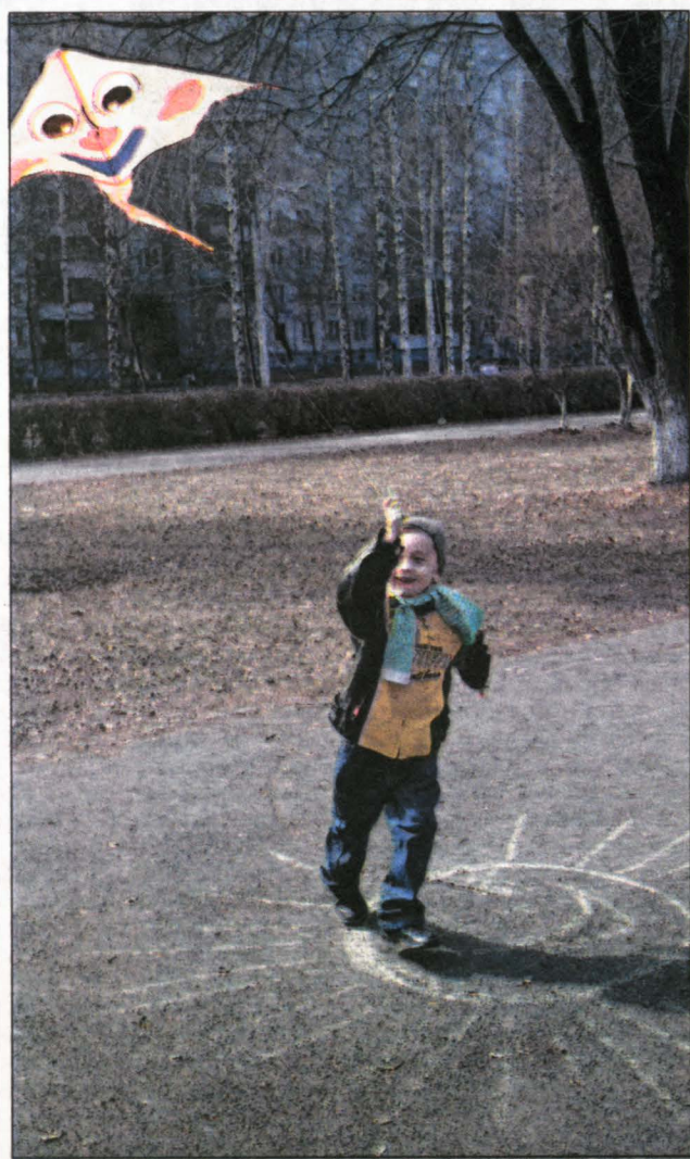
«Солнечная активность».
