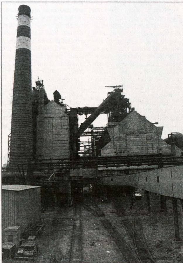
Доменная печь №3 на ЗСМК после остановки была запущена летом. Теперь все три домны Запсиба работают еще и на НКМК.
