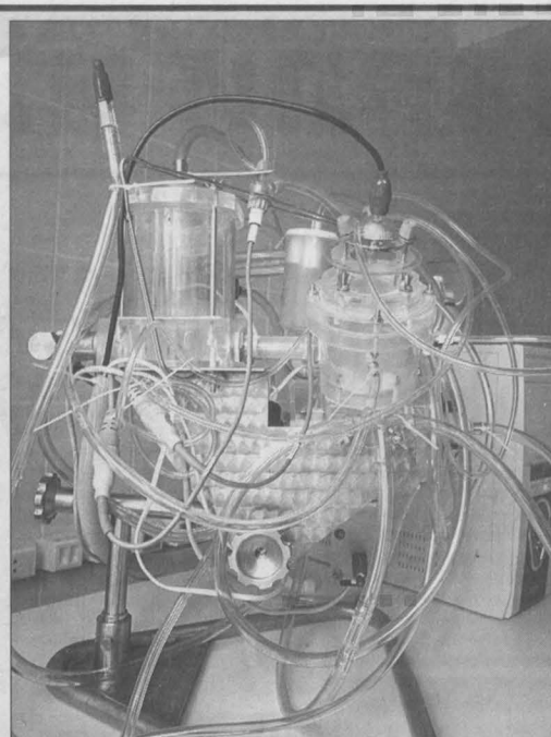
Стенд для гидродинамических исследований биопротезов клапанов сердца.
