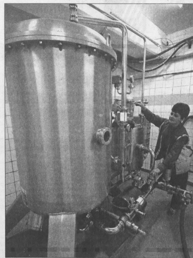
Кизельгуровый фильтр для пива. Саликова Лариса Ивановна, оператор производства пищевых продуктов.
