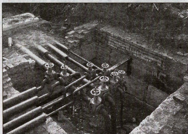
Трубы, утепленные пенополиуретаном.
