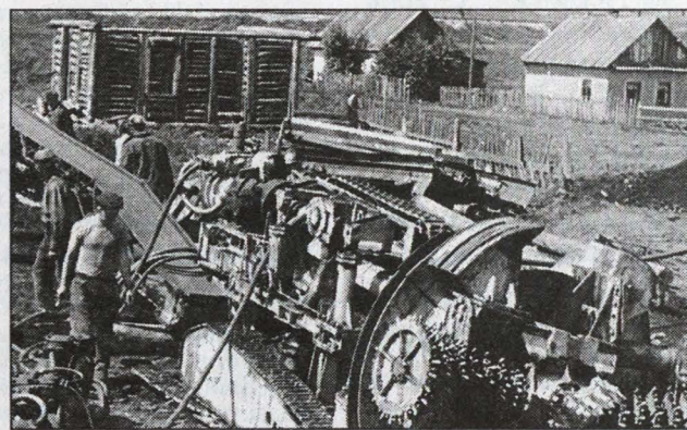
Комбайн Гуменика (ПКГ), сконструированный механиком шахты «Байдаевская» Яковом Яковлевичем Гумеником (1920-1995), в годы пятой пятилетки позволил удвоить добычу угля на шахтах треста «Куйбышевуголь».
