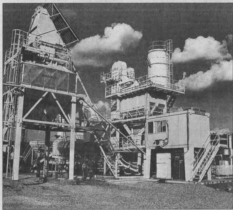
Дробильно-сортировочный комплекс.
