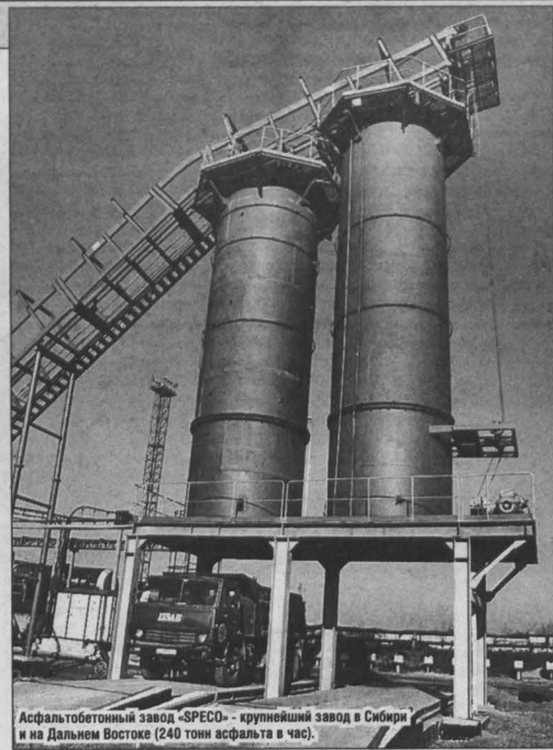
Асфальтобетонный завод «СПЕКО» — крупнейший завод в Сибири и на Дальнем Востоке (240 тонн асфальта в час)
