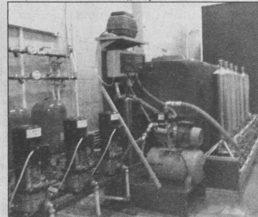
Станция комплексной очистки воды «Ручей-4М».
