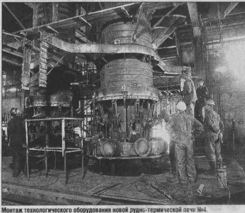
Монтаж технологического оборудования новой рудно-термической печи №4.
