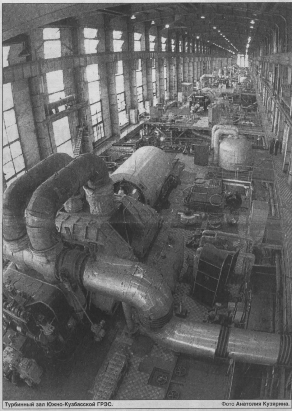
Турбинный зал Южно-Кузбасской ГРЭС.
