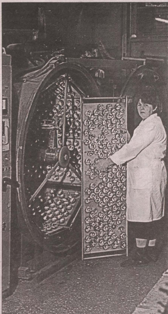
Вакуумное напыление алюминием на отражатели.
