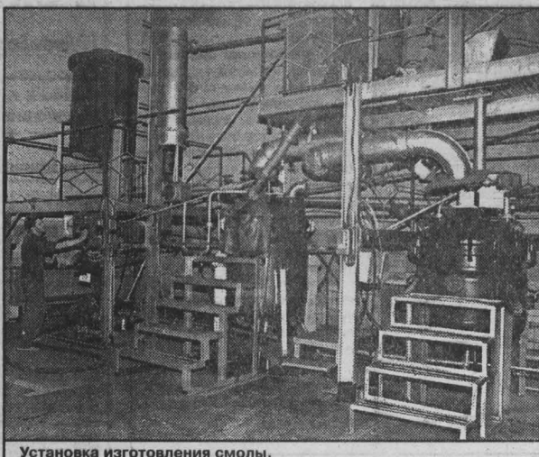
Установка изготовления смолы.
