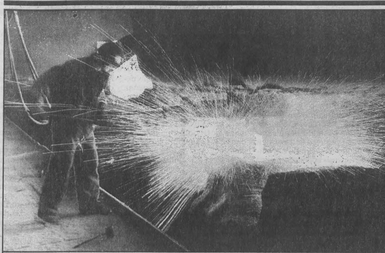
Разливка стали.
