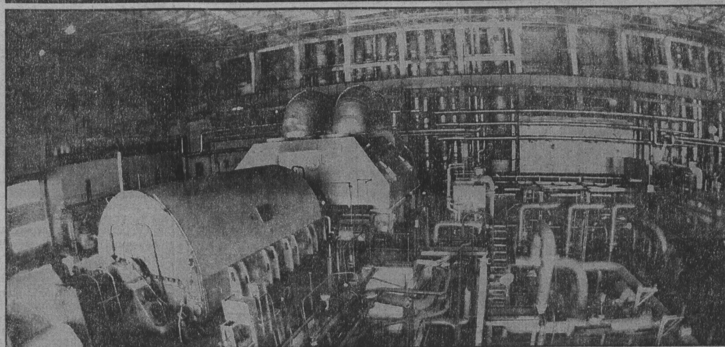
Турбинный зал Беловской ГРЭС.
