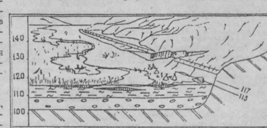
Палеоландшафт окрестностей Писаной периода завершения накопления озерно-речных и болотных отложений верхней поймы, средний голоцен (6 тыс. лет назад).
