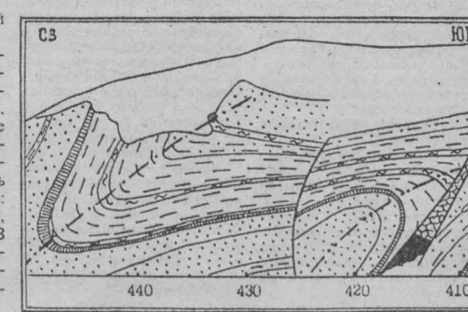
Береговой геологический разрез скалы Писаной: 1 — песчаники, 2 — алевролиты, 3 — глинистые сланцы, 4 — разрывные нарушения, 5 — рифовый известняк.
