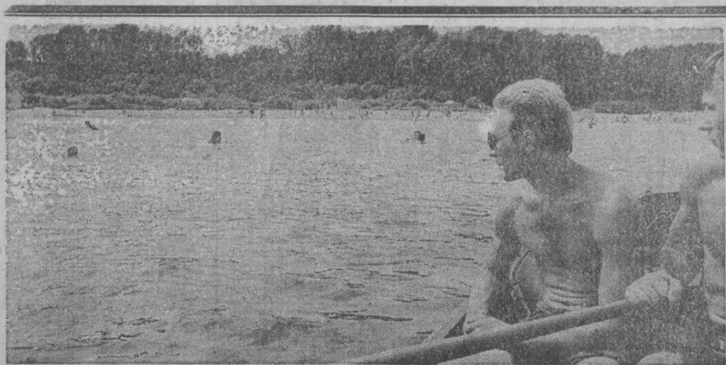
проблема лета
