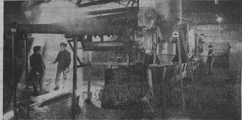
Новый кормоцех сдан в постоянную эксплуатацию для животноводов госплемзавода «Ленинск-Кузнецкий». Серийный агрегат КОРК-15 полностью переделан, значительно повышена его производительность. Нормы сдвигаются микроэлементами, смешиваются и измельчаются.
