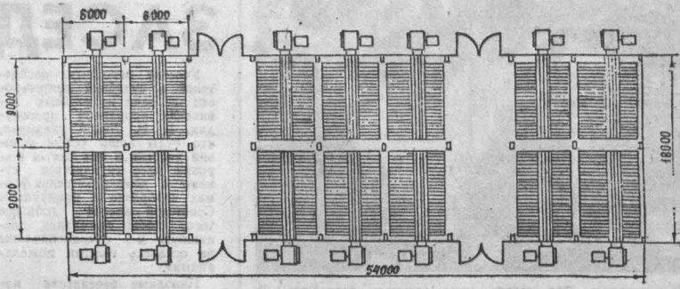
Схема установок активного вентилирования прямоугольного типа.
