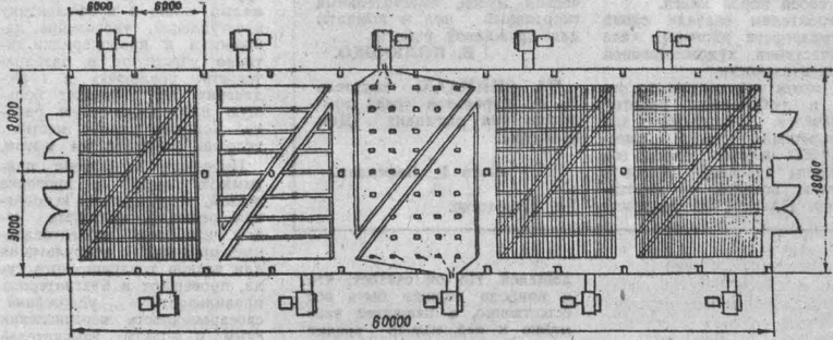
Схема установок активного вентилирования диагонального типа.
