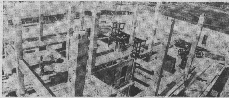
Продолжается строительство многоэтажной гостиницы «Турист». Монтаж каркаса здания осуществляет бригада Николая Дмитриевича Марченко из СУ-2 треста «Кемеровогражданстрой». Этот коллектив обязался до конца года полностью завершить монтажные работы. НА СНИМКАХ: бригадир Н. Д. Марченко; идет монтаж деталей на четвертом этаже гостиницы. Фото В. Грызыхина, г. Кемерово.
