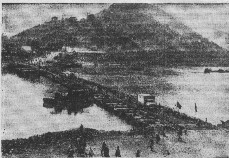
СРВ. По всей республике раскинулись объекты советско-азиатского экономического сотрудничества. Недавно вступил в строй понтонный мост на Черной реке (на снимке), где ведется сооружение крупнейшего в стране гидроузла Хоабинь. Новый мост позволит в значительной мере повысить эффективность работы транспорта на главной стройке республики, будет способствовать успешному выполнению графика работ.
