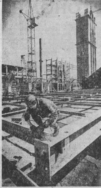
Верхолазы — стальмон. тажины кемеровского управления «Сибсталь» — на стройке приходят к своим из первых. От их работы, их мастерства зависит в не малой степени прочность и долговечность корпусов и сооружений новых химических производств.
