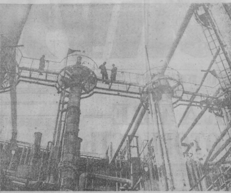
67 процентов продукции со Знаком качества выпускают трудящиеся объединения «Азот». НА СНИМКЕ: один из технологических узлов производства нитратам-2. Фото Ю. Сергеева.
