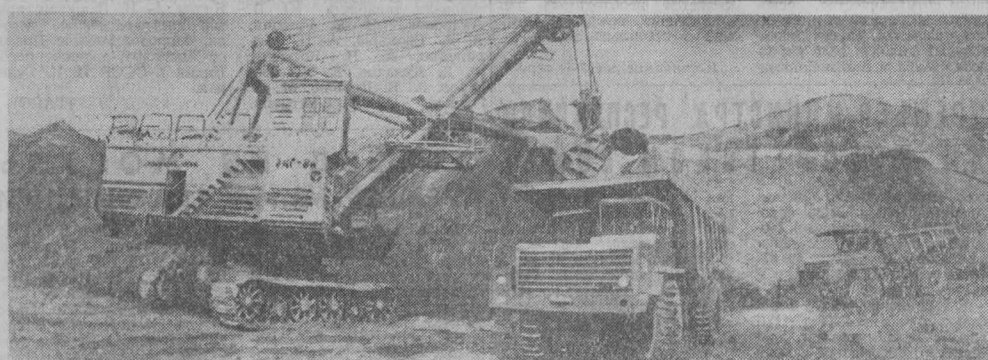
РАЗРЕЗ «Кедровский» вступил в строй действующих угольных предприятий Кузбасса в начале 1955 года. За 23 года существования разреза добыча угля на нем возросла в четыре раза, объем вскрышных работ — в пятнадцать раз, производительность списочного экскаватора — в четыре раза. НА СНИМКЕ: в забое разреза «Кедровский». Фото Ю. Сергеева.
