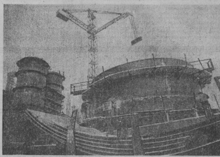
На Западно-Сибирском металлургическом заводе идет реконструкция первой доменной печи. Комсомольско-молодежная бригада монтажников Василия Архипова из первого Новокузнецкого монтажного управления ведет здесь монтаж здания и блока воздухогревателей. Вместе с монтажниками трудятся на реконструкции и ведущая бригада этого управления, возглавляемая Иваном Цивилевым. Ежемесячно
