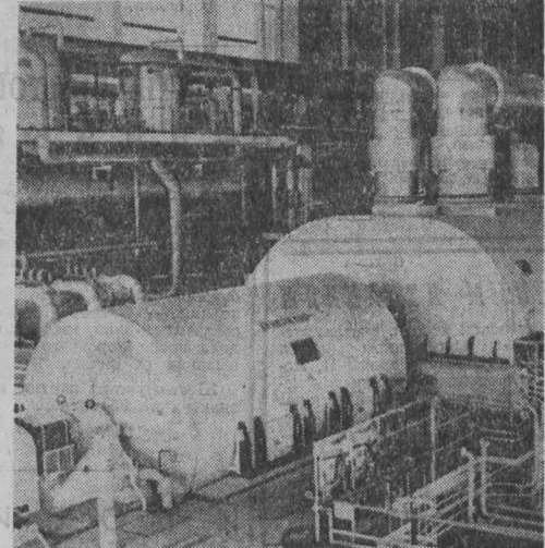
Накануне 30-летия социалистической революции в Болгарии была торжественно введена в действие первый блок атомной электростанции «Козлодуй», строящейся при техническом содействии Советского Союза. НА СНИМКЕ: в машинном зале АЭС. Фото БТА-АПН.
