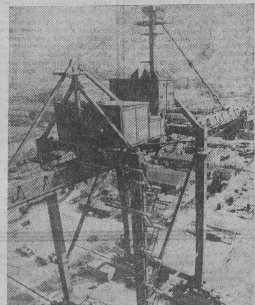
Германская демократическая республика. В рамках СЭВ завод «ФТА» в Лейпциге специализируется на производстве мощных кранов для разгрузки контейнеров весом 10, 20, и 30 тонн. НА СНИМКЕ: кран, изготавливаемый по заказу Советского Союза. Фото ЦВ-АПН.
