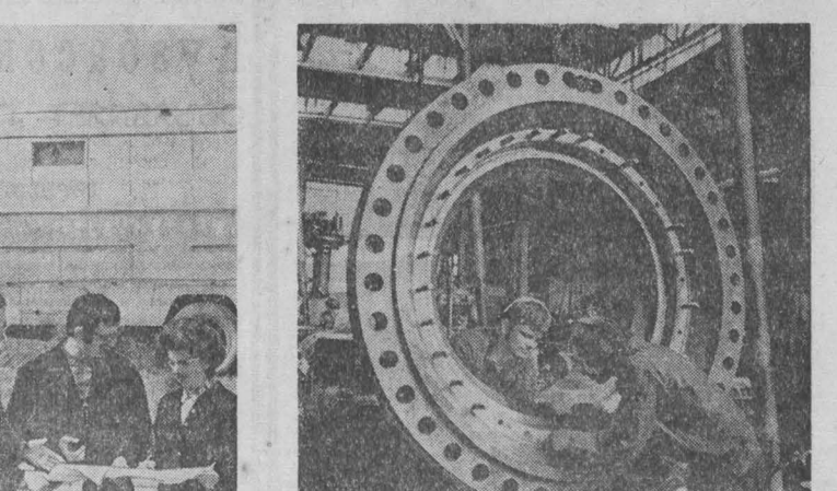
Завод монтажного оборудования в Долне-Бенешове (Советская Чехословакия) выполняет крупный заказ Советского Союза на оборудование для строящегося в Сибири газопровода. В частности, здесь изготавливают сферические клапаны. На снимке: монтаж клапана диаметром 1.000 мм для Советского Союза.
