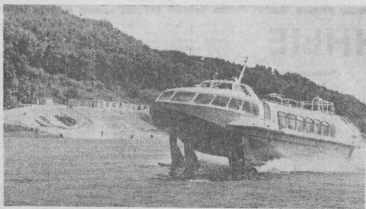
ГОРЬКИЙ «Восток-2» — судно, пополнившее семейство «крылатого флота». Этот новый корабль, которому предстоит заменить «Ракету», спроектирован в ЦКБ по судам на подводных крыльях...
