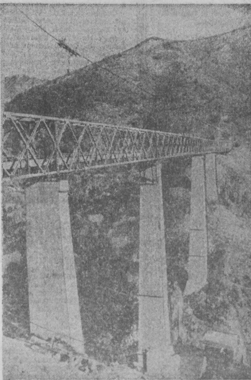
СФРЮ. Через каньон Малой Риены в Черногории возведен самый высокий в Европе мост (на снимке). Его опоры поднялись на высоту 223 метров. Это уникальное сооружение является частью строящейся железнодорожной магистрали Белград — Бар.
