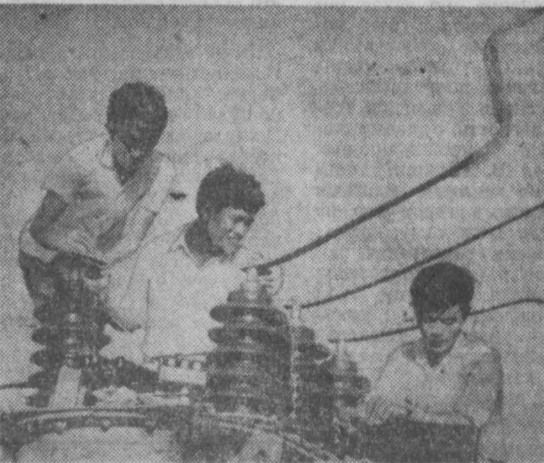
Правительство ДРВ на ближайшие три года наметило широкую работу по совершенствованию гидротехнических систем. НА СНИМКЕ: проверка восстановленного электробоорудования на насосной станции, подающей воду на поля. Фото БНА—ТАСС.
