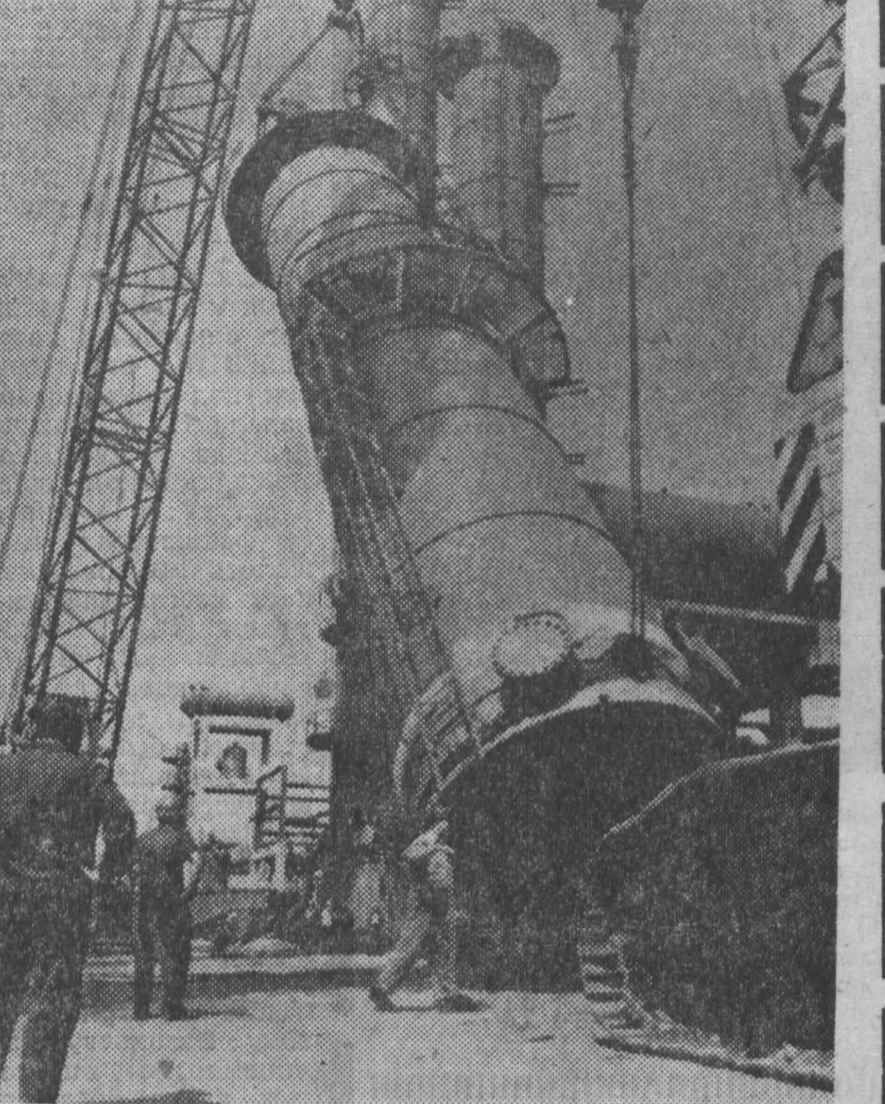
НА СНИМКЕ: установка ректификационной колонны на строительстве завода.
